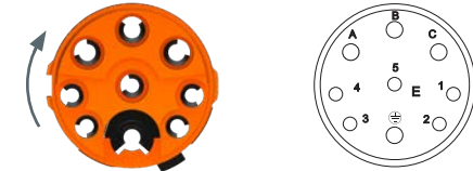
Ansicht steckseitig
