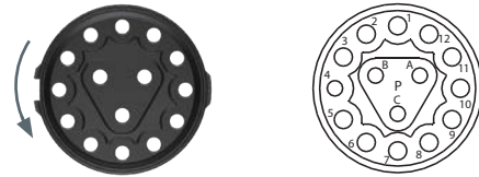
Ansicht steckseitig
