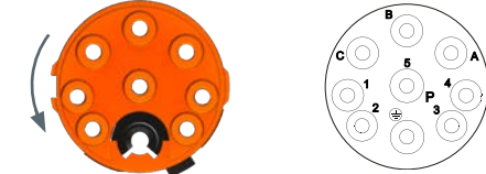
Ansicht steckseitig
