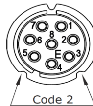
Polbild / pin arrangement Ansicht steckseitig / view mating side
