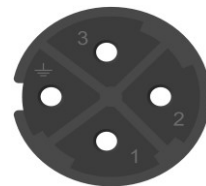
Polbild / pin arrangement Ansicht steckseitig / view mating side
